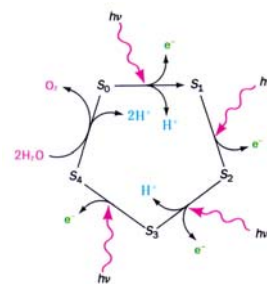
光化学系IIの酸素発生反応過程を時間ごとに追ってプロセス解明を目指す
