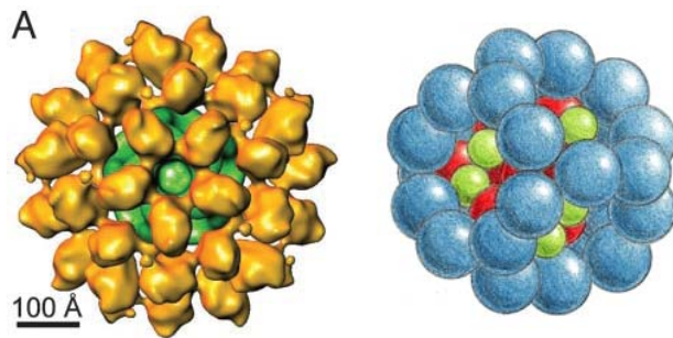
ビルビン酸脱水素酵素の電子顕微鏡単粒子解析による構造(左)とその模式図(右)。ウイルスだけでなく、このように繰り返し構造を持った超分子複合体は多く生体中に存在する。これらがSACLAのターゲットとなる。
