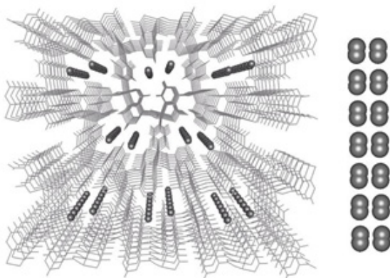
気体吸着素子の動的機構解析に期待 (整列酸素分子を細孔に持つ[Cu(pydc)2(pydz)2]の結晶構造)
