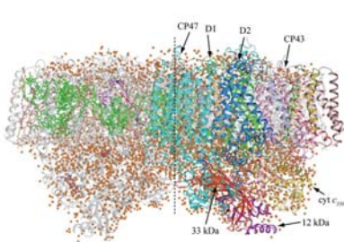
光化学系IIの1.9 Å分解能の構造(Umena, Y. et al. Nature 2011)。日本で解析されかつ本課題に適した蛋白質の例。
